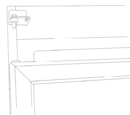
6. Monter le pivot de la charnière dans le côté contraire sans le tendre.
